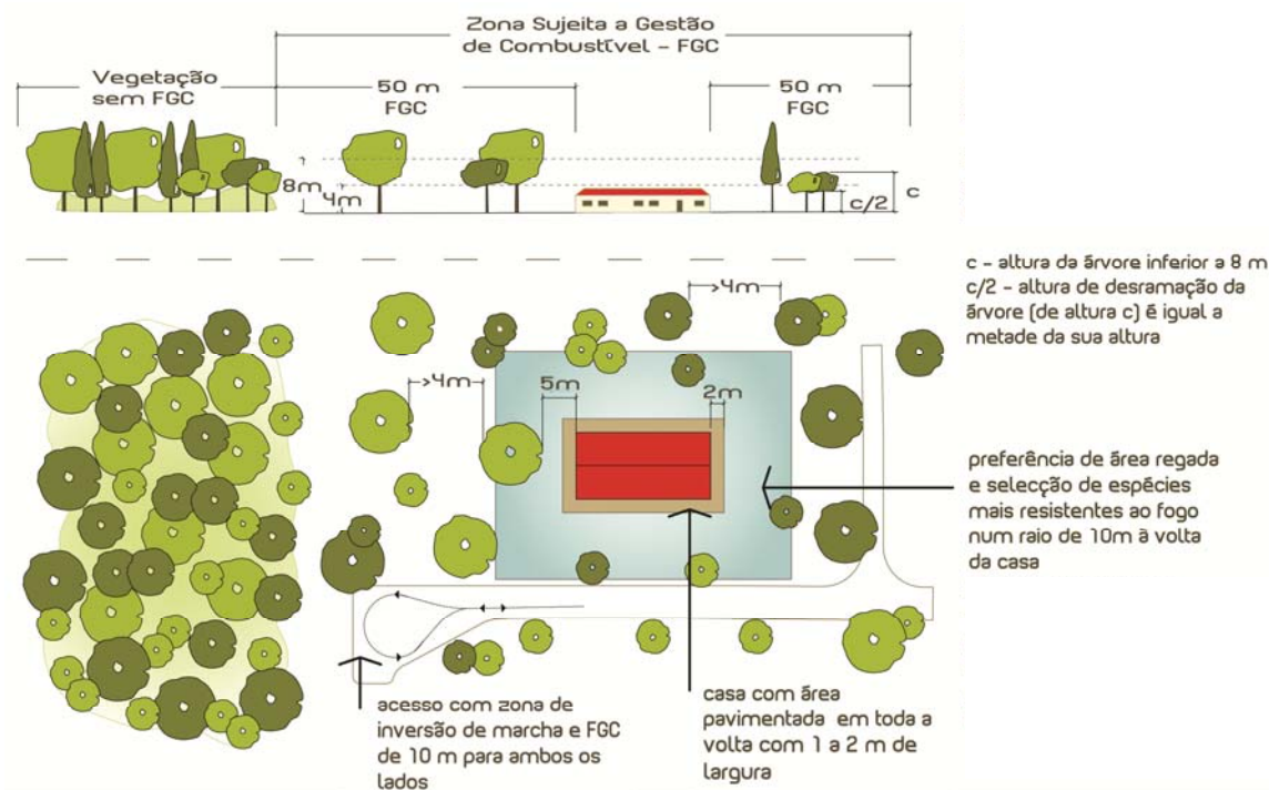
Figura 14 - Esquema exemplificativo da implementação de uma Faixa de Gestão de Combustíveis à volta de uma edificação. A - esquema com vista frontal; B - esquema com vista em planta.
