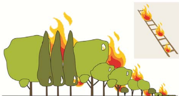
Figura 8 - Esquema representativo da evolução de um incêndio ao longo dos estratos herbáceo, arbustivo e arbóreo.
